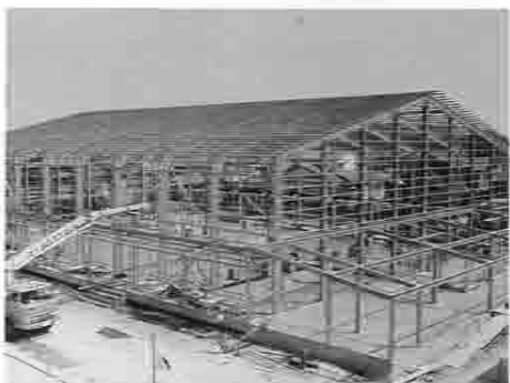
体育館建築
